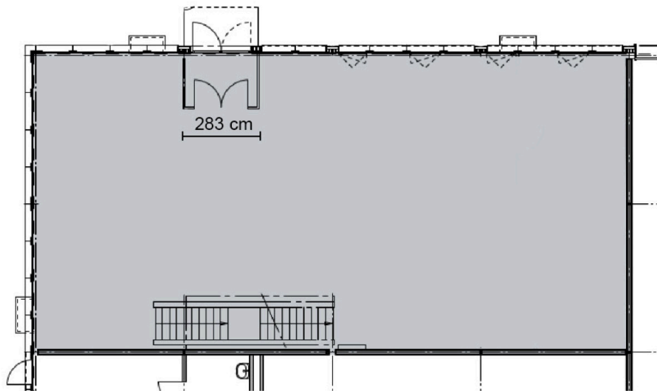
Grundriss Erdgeschoss
